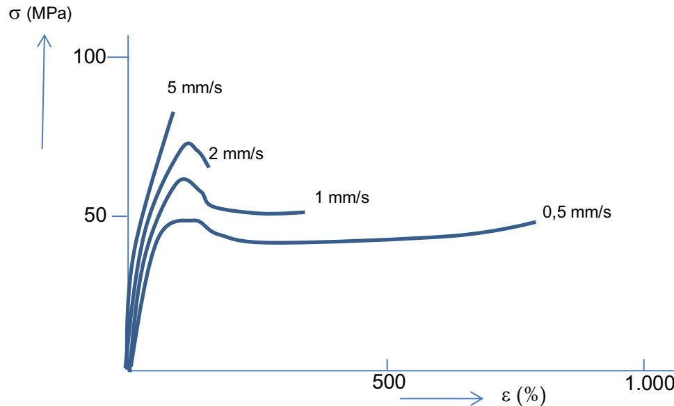
Figuur 26.6: Invloed van de deformatsiesnelheid op het spanning-rekdiagram van een kunststof
