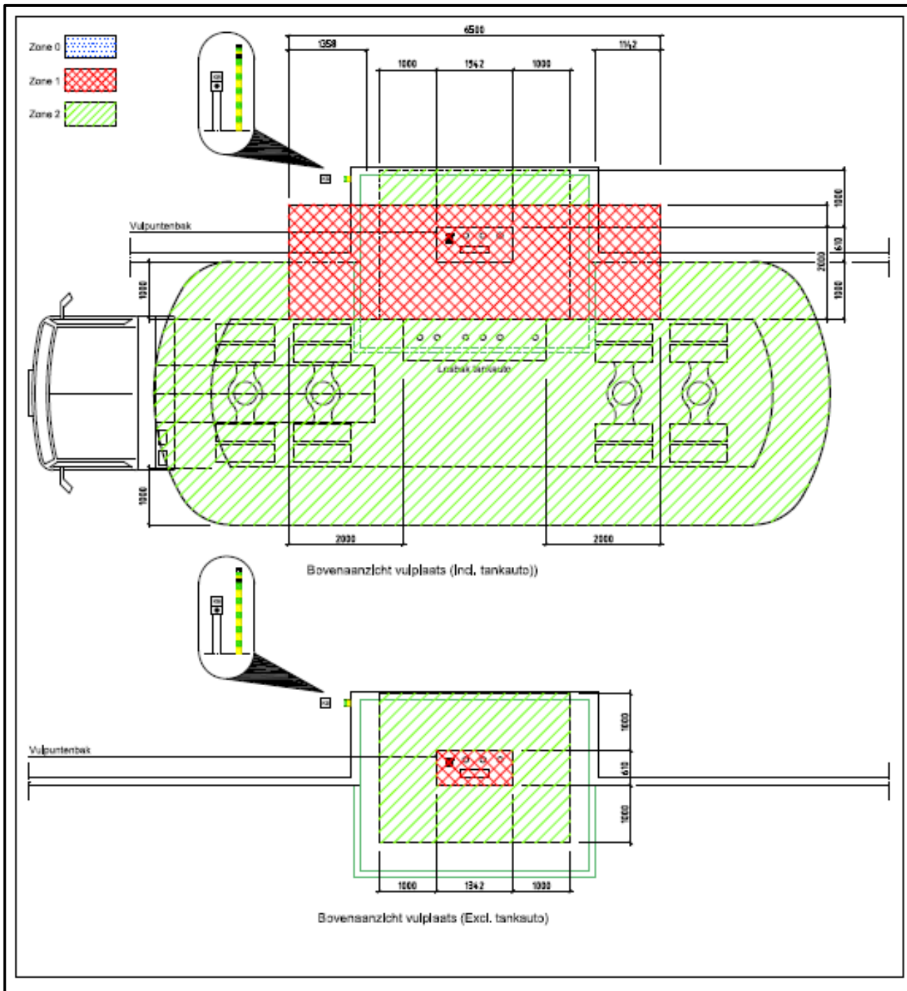
Figuur VI.5.1 – Voorbeeld van zonering vulpuntmorsbak – bovenaanzicht vulplaats
