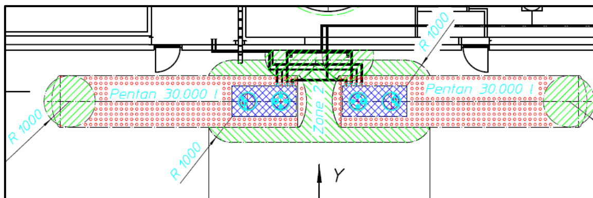
Figuur VI.6 – Voorbeeld van Ondergrondse pentaantanks (bovenaanzicht)
